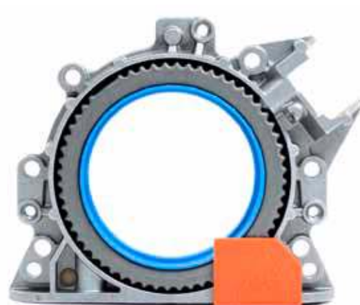
Ilustracja 1_Zintegrowany pierścień uszczelniający wał
